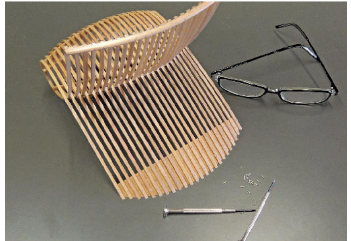
/ Mit 168 Linsenkopfschrauben im Durchmesser von knapp 1 mm sind die einzelnen Schleifen aus Buche untereinander und mit den Querstreben verbunden.
